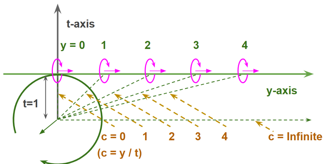
図3-6. 傾き(速度)に応じてR-spaceが投影された空間座標を進む回転ベクトル
