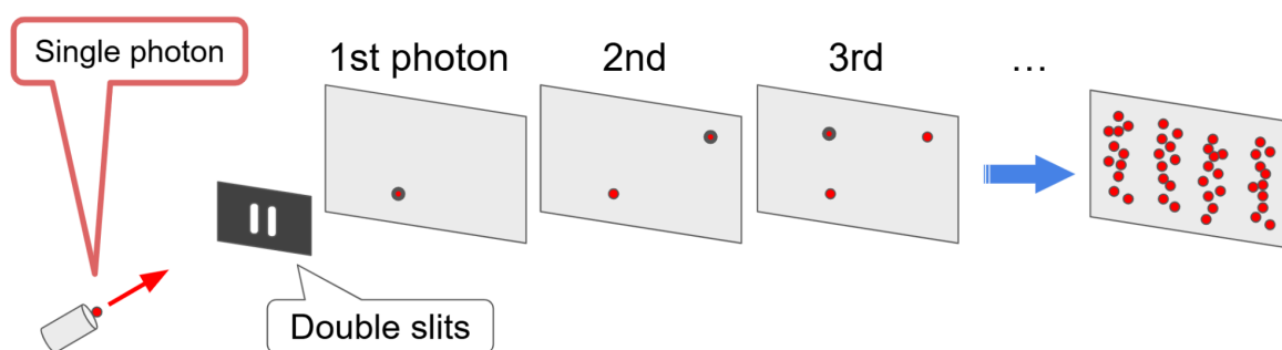
図2-2. 量子の2重スリット実験
