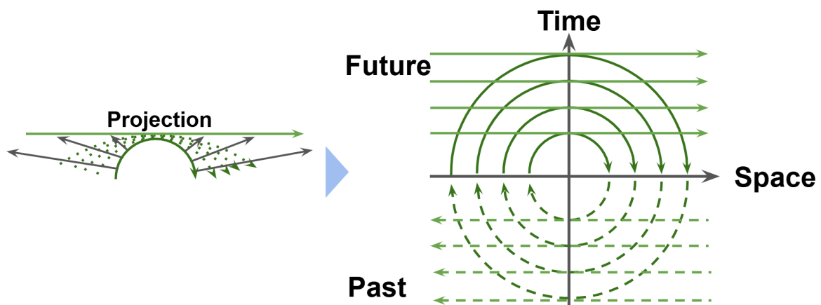
図3-4. R-spaceの時空間への投影
